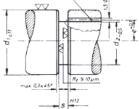
Entlüftungsbohrung druckseitig bei Bedarf
